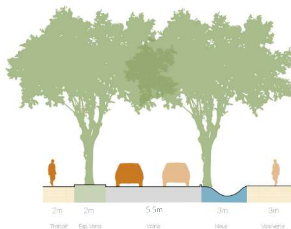
Principe voie principale - 15.5m
