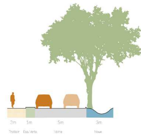
Principe voie secondaire - 11m
